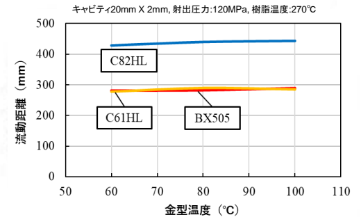
■金型温度と流動距離
