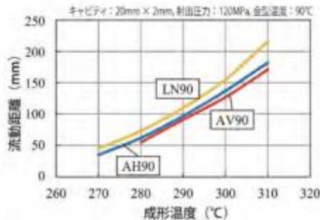
■樹脂温度と流動距離
