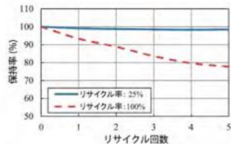
■ GH30 のリサイクルによる曲げ強さの保持率
