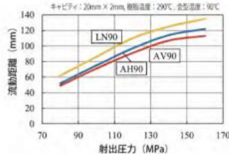
■射出圧力と流動距離
