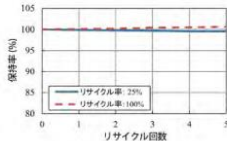
■ LN80 のリサイクルによる引張強さの保持率
