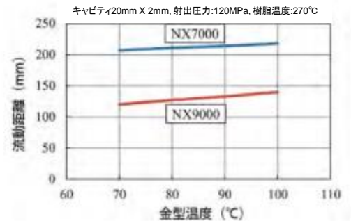
■金型温度と流動距離
