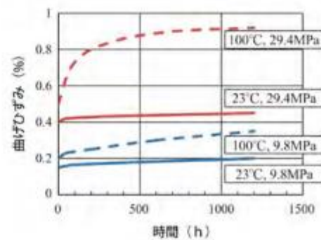
■GH30の曲げクリープ特性
