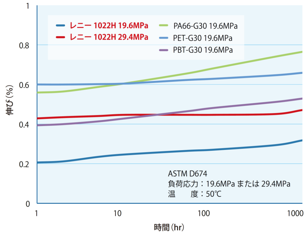
■ 引張クリープ
