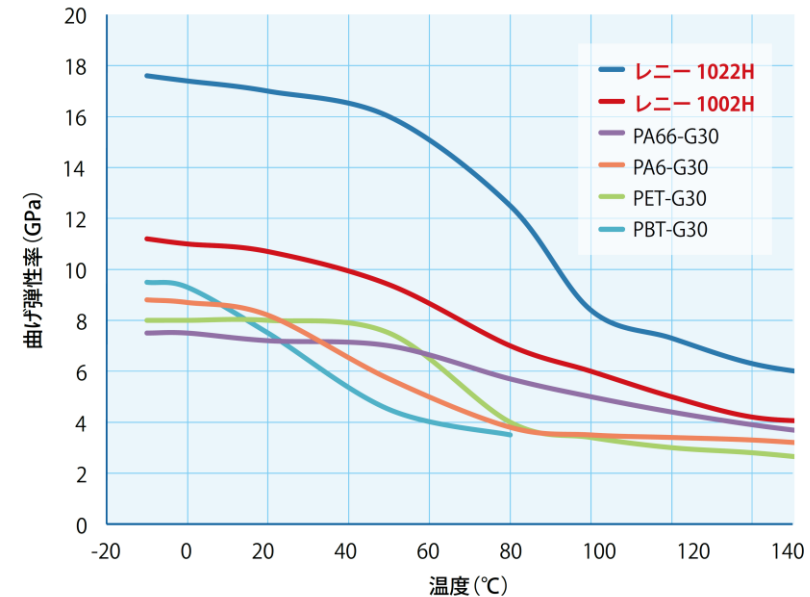
図2 曲げ弾性率 温度依存
