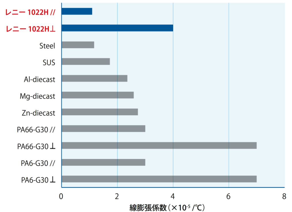
■ 線膨張係数の比較
