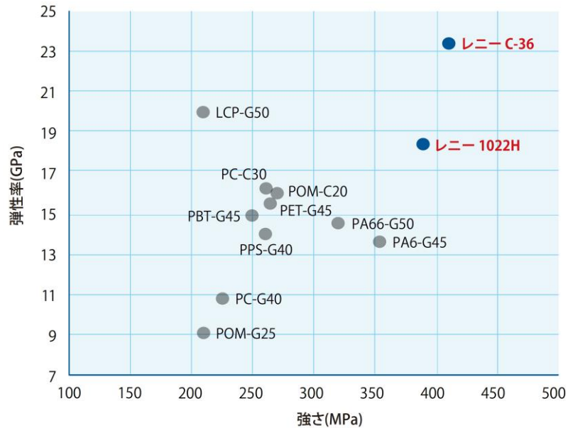
図1 曲げ強さ 曲げ弾性率(乾燥試験片)
