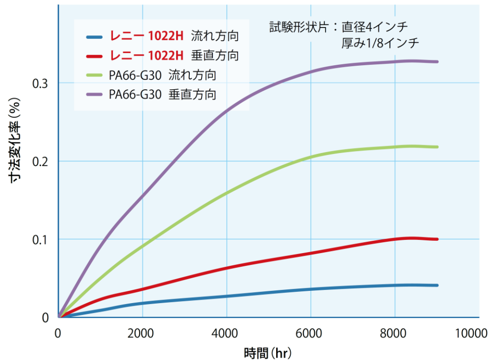
■ 20°C/65%RHにおける寸法変化
