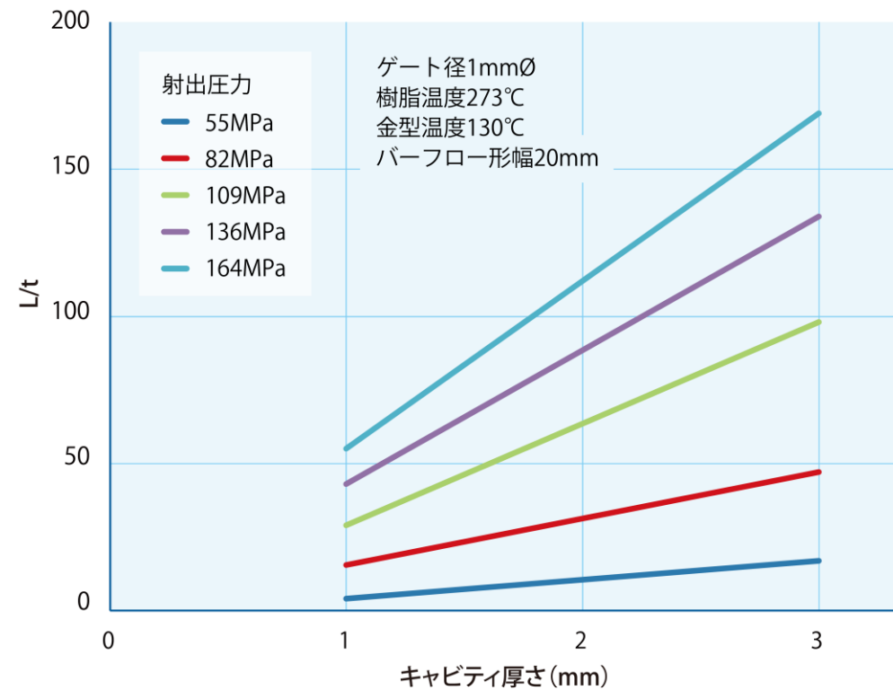
■ レニー 1022Hのキャビティ厚さと L/t
